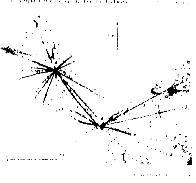
La foto probabilmente impressionata dall'antiprotone nel gennaio del 1955, e archiviata alla descrizione pubblicata dai professori Amaldi, Castagnoli, Corini, Franzoni e Mantrelli sul "Nuovo Cimento"
