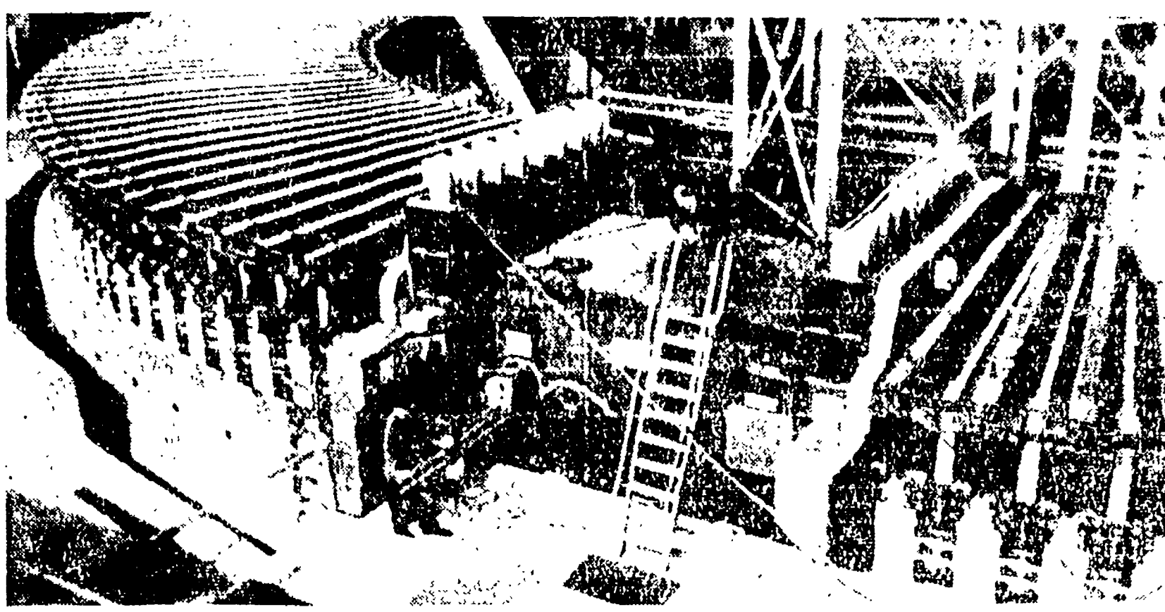
Una visione parziale del bevatrone di Berkeley, in California.
