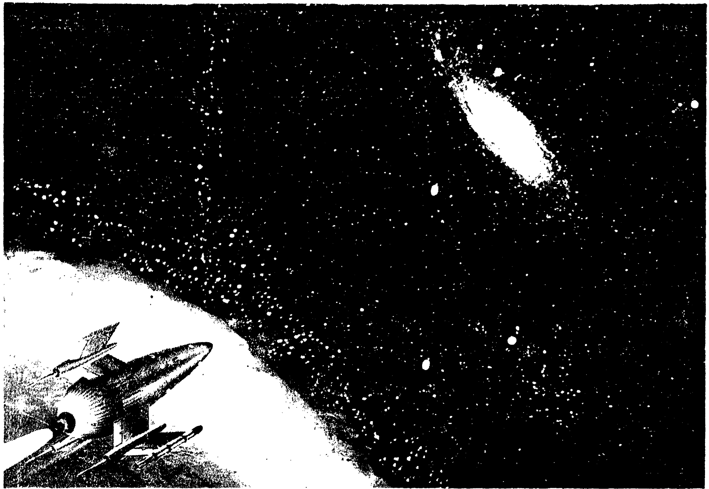
...Operazio che collaborò a fabbricare i metalli che resero possibili i viaggi spaziali fino alla periferia della nebulosa Andromeda. Nel fotomontaggio la nebulosa Andromeda ripresa attraverso il telescopio di Mount Wilson
