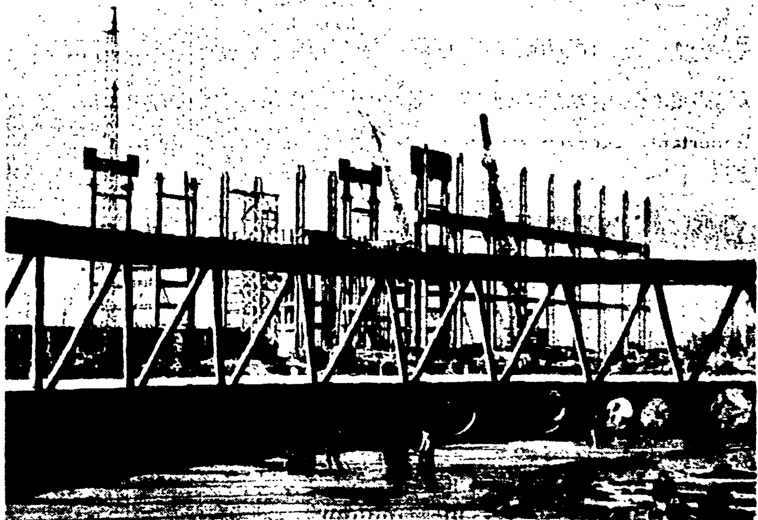
POLONIA. La nuova centrale idroelettrica in costruzione a Turaszyn.
