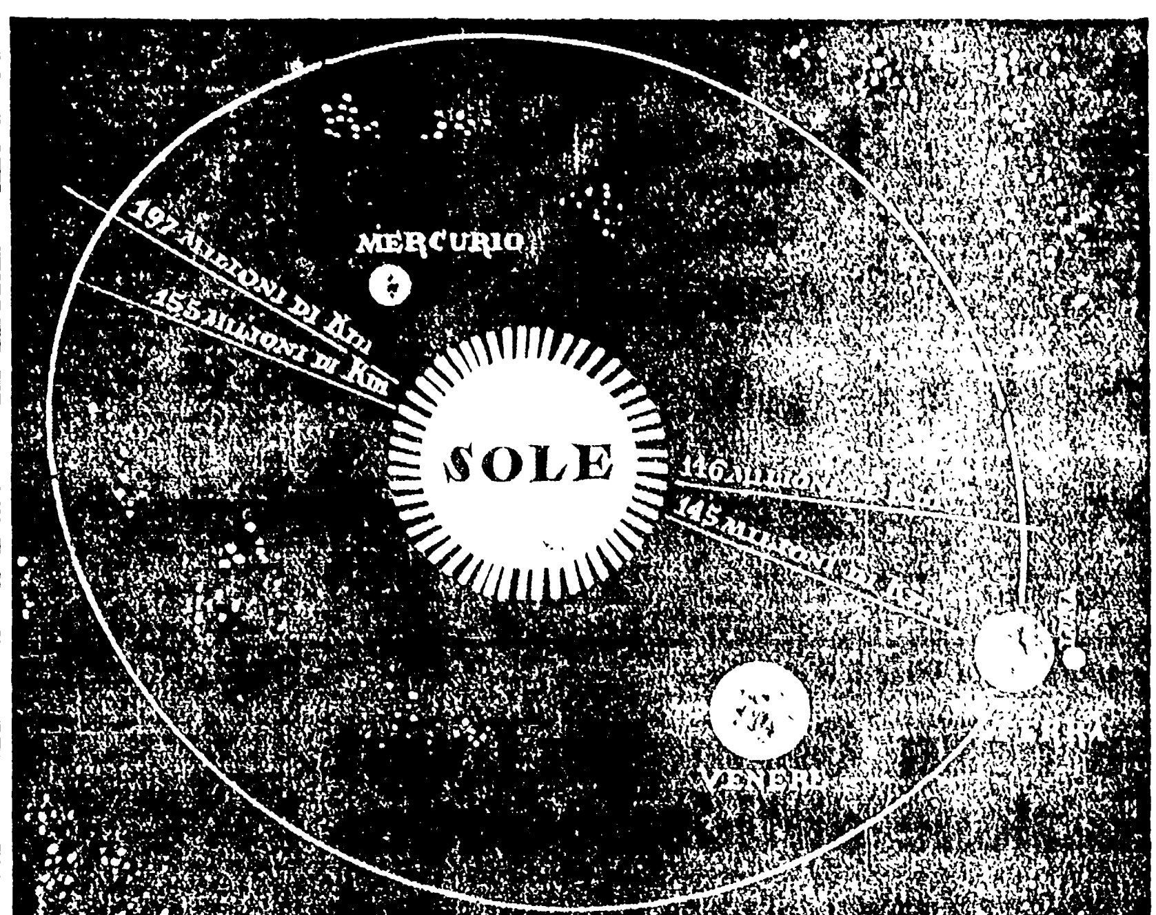
La posizione di alcuni pianeti (Terra, Venere, Mercurio) rispetto al Sole
