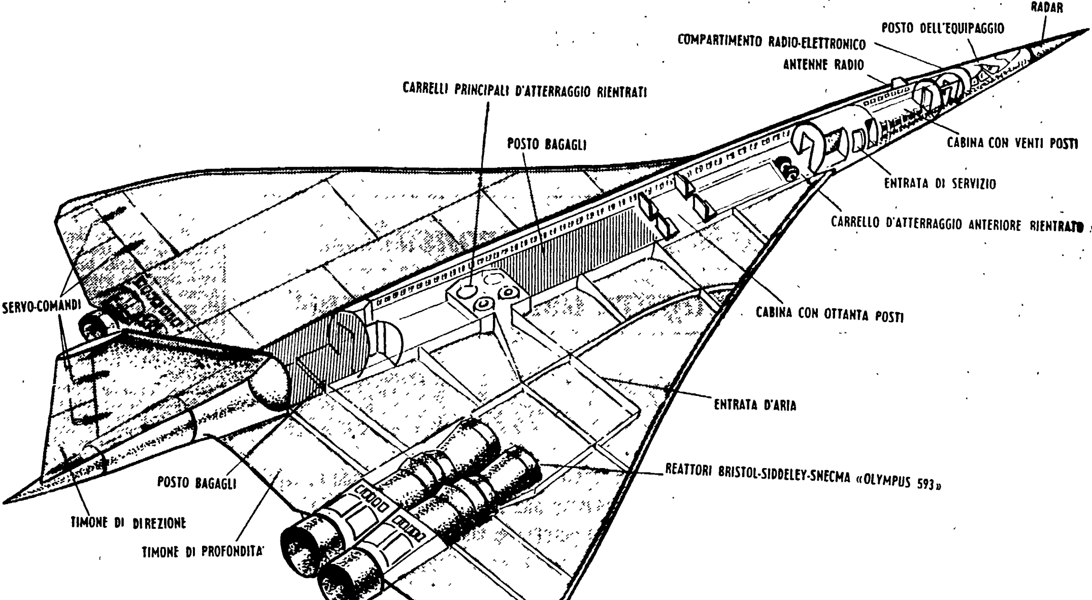
Schema di un «Concorde»
