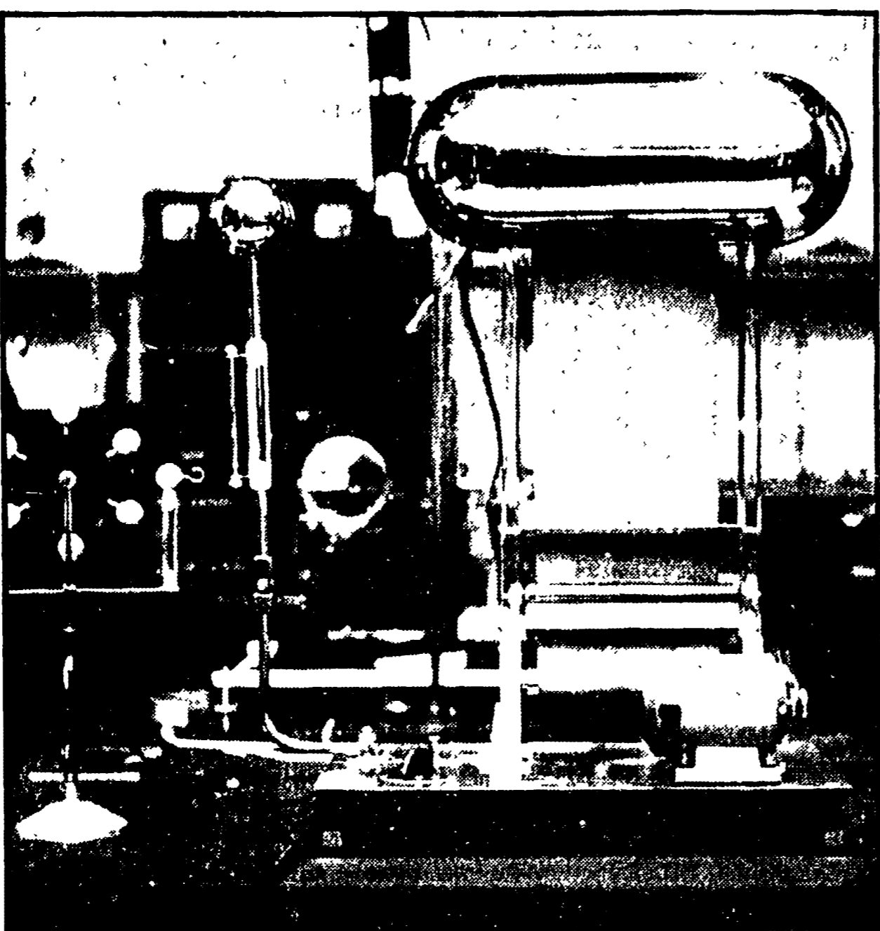
Macchina elettrostatica a strofinio mediante la quale si possono ottenere scariche ad alta tensione, caricare condensatori e provocare scariche nei tubi a gas rarefatti. Nella foto in testata: banco fotografico per lo studio dei fenomeni inerenti le lenti e l'intensità dei raggi di luce.
