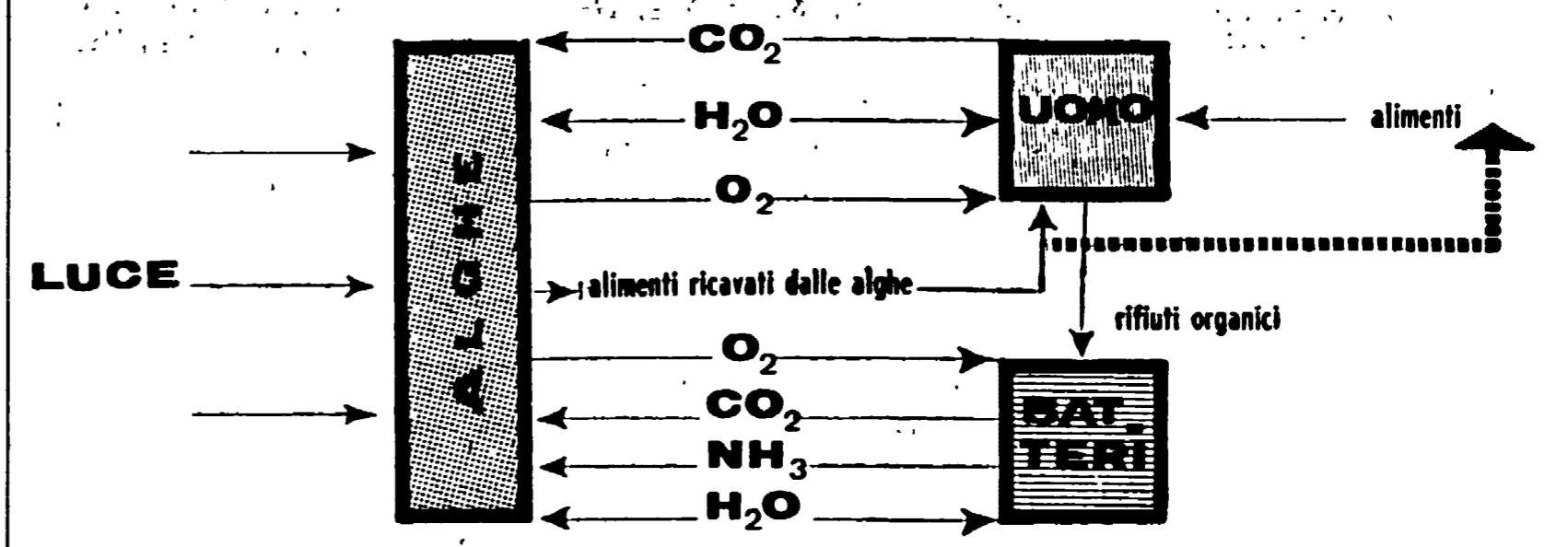
Recupero biologico dei calcoli (rifiuti) organici secondo Oswald e Goineke, dei laboratori Leeds e Northrup. Velocità di trasformazione: da 20 a 30 volte superiore a quella normale (agricola). Peso dell'attrezzatura: 150/200 Kg. pro capite
