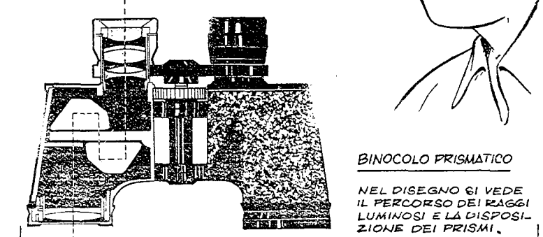
NEL DISEGNO SI VEDE IL PERCORSO DEI RAGGI LUMINOSI E LA DISPOSIZIONE DEI PRISMI.
