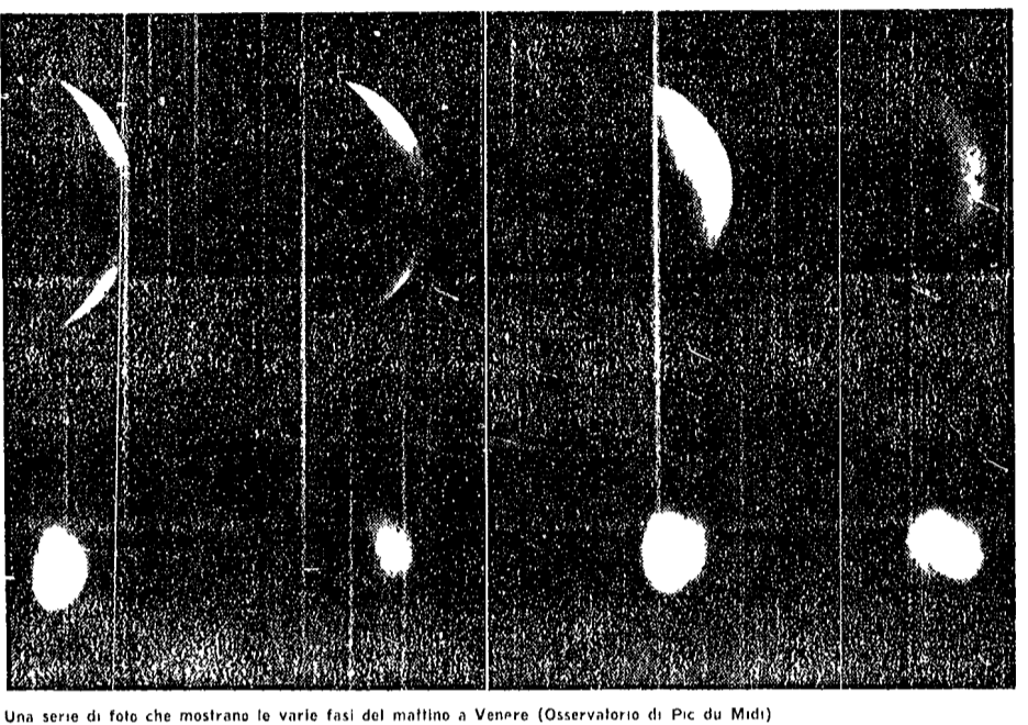
Una serie di foto che mostrano le varie fasi del mattino a Venere (Osservatorio di Pic du Midi)
