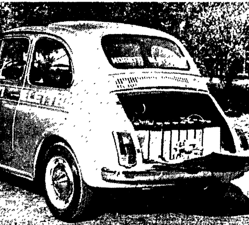
La Fiat 500 con il motore elettrico messo a punto dalla Moratti di Torino. Il motore, alimentato da batterie a 36 elementi, sviluppa una potenza di 3 HP ed una velocità di 35 km./ora. L'autonomia è di 100 chilometri. Per ricaricare le batterie sono necessarie da 8 a 10 ore.
