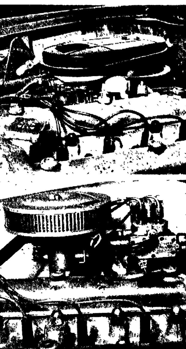
Nella foto in alto: come si presenta il vano motore della Giulia 1300 TI di serie; nella foto in basso: il vano motore con l'apparato dell'ing. Mastropaulo.
