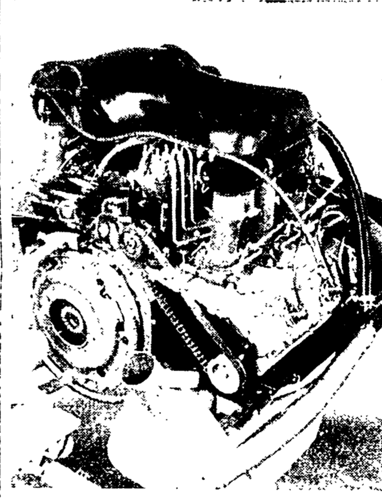
Il motore ad iniezione della Porsche in primo piano è visibile la cinghia dentata della Uniroyal.
