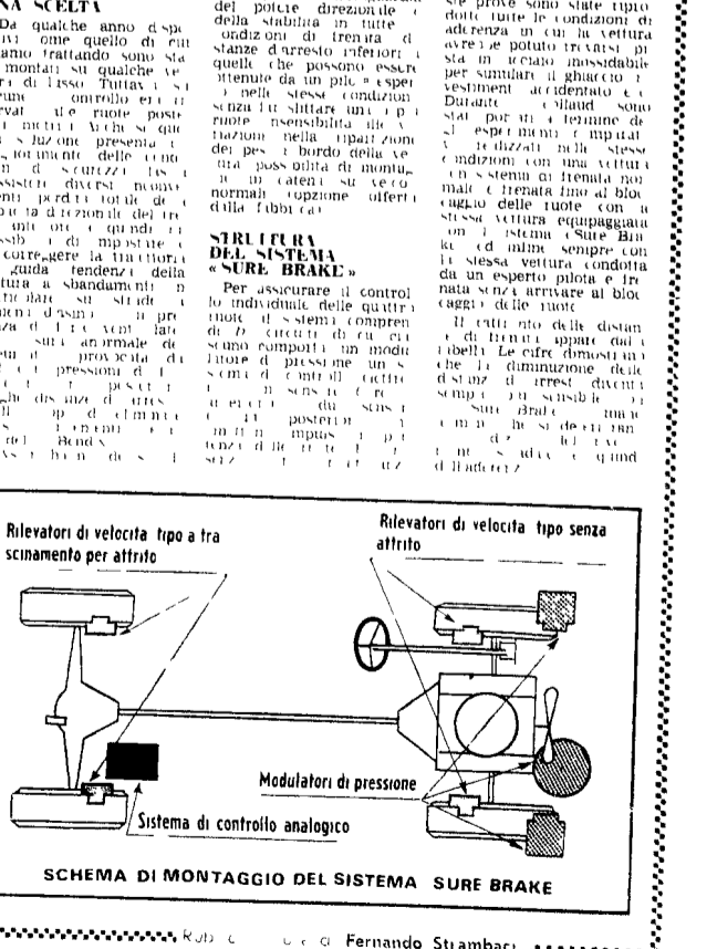
SCHEMA DI MONTAGGIO DEL SISTEMA SURE BRAKE
