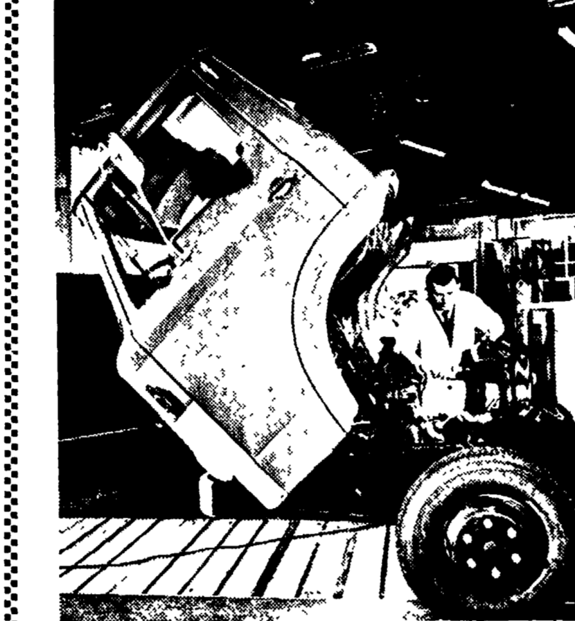
Una delle singolari caratteristiche degli autocarri Ford «D» è data dalla possibilità di ribaltare la cabina...
