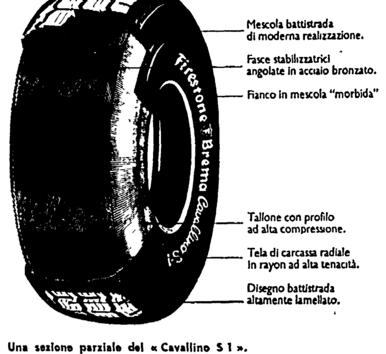
Una sezione parziale del «Cavallino S1».
