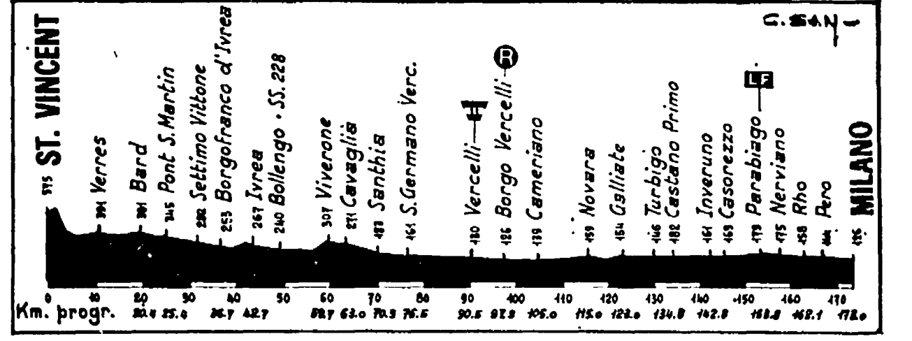
L'altimetria della tappa oderna St. Vincent-Milano
