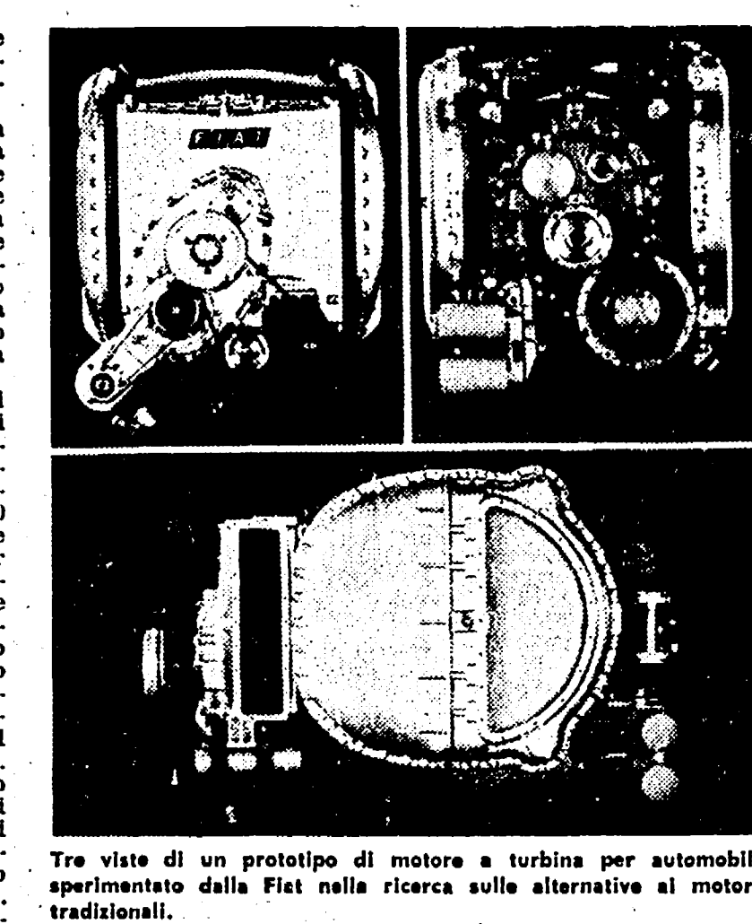
Tre viste di un prototipo di motore a turbina per automobili sperimentato dalla Fiat nella ricerca sulle alternative ai motori tradizionali.
