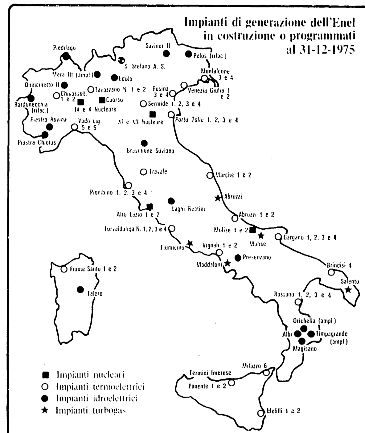
La cartina indica la localizzazione degli insediamenti programmati nel 1975 dall'ENEL nei settori nucleare, termoelettrico, idroelettrico e turbogas...
