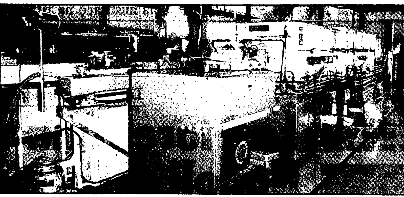
Un particolare dei forni di sintesi per l'arricchimento dell'uranio nella centrale di Bosco Marengo (Alessandria).
