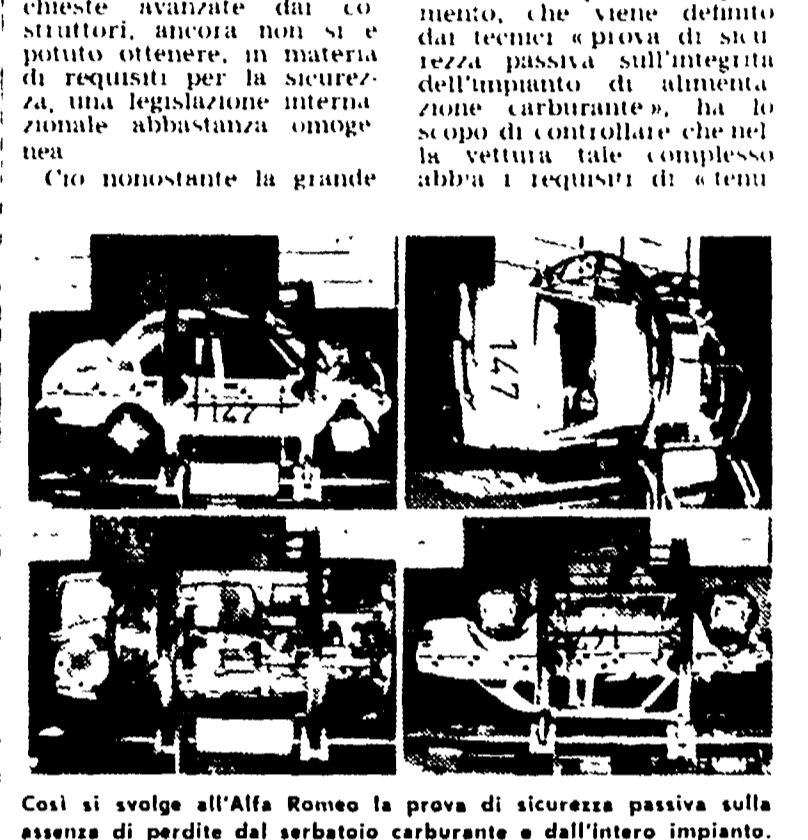
Così si svolge all'Alfa Romeo la prova di sicurezza passiva sulla assente di perdite dal serbatoio carburante e dall'intero impianto.
