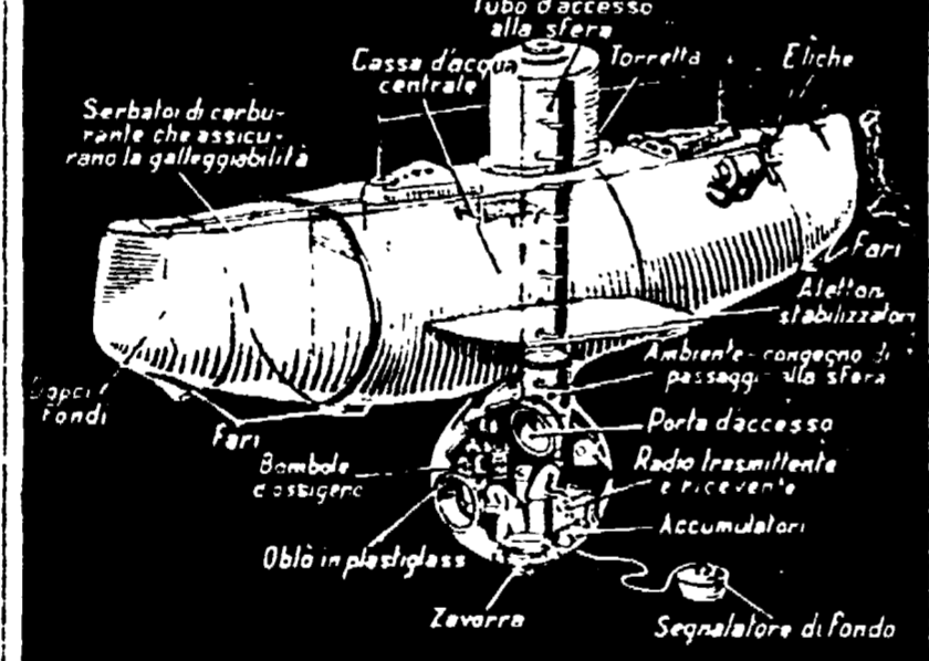
Ecco, in uno schema accurato, il batiscavo di Piccard, che compie le sue esperienze nel mare di Ponza
