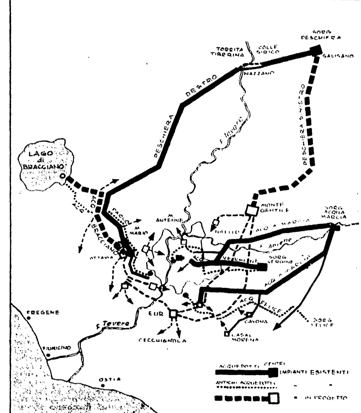
L'ACQUA DI ROMA — Lo schema degli impianti ideati di approvvigionamento e di adduzione. Le linee unite rappresentano gli impianti esistenti, quelle punteggiate gli antichi acquedotti, quelle tratteggiate gli impianti progettati
