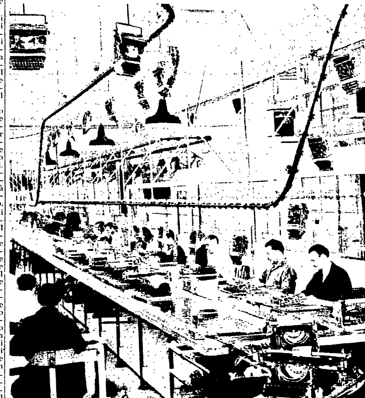
Olivetti reparto del collaudo meccanico. Nella parte sinistra si collaudano le macchine standard che arrivano sul trasportatore a rulli e passano a un trasportatore a nastro che scorre davanti al loro posto.
