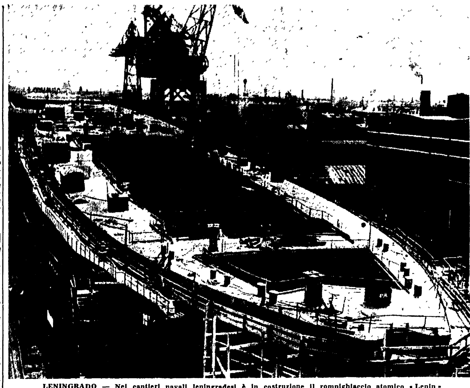
LENINGRADO - Nel cantiere navale leningradese è in costruzione il rompighiaccio atomico «Lenin»
