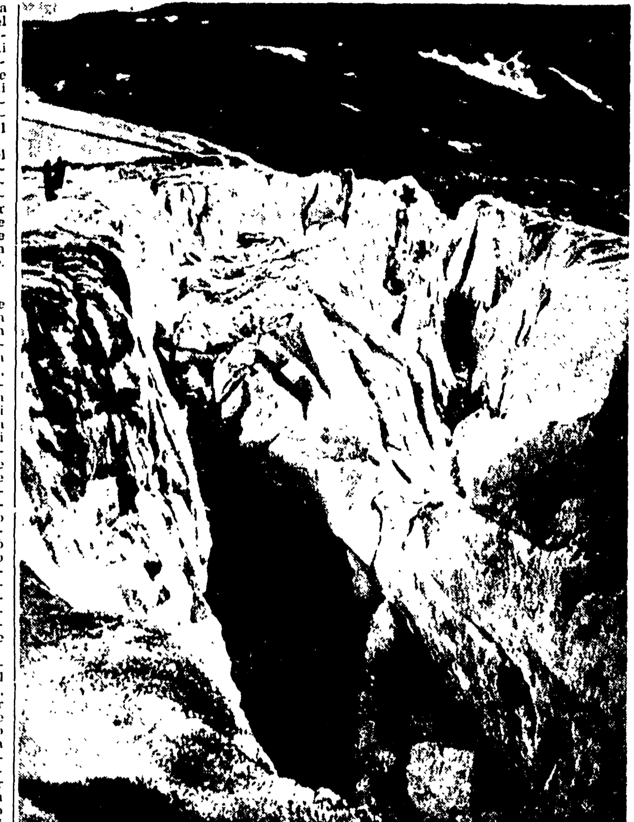
VALLE D'AOSTA - Il diaframma di un crepaccio corrotto per lo stramento degli strati inferiori nel Ghiacciaio del Rutor.
