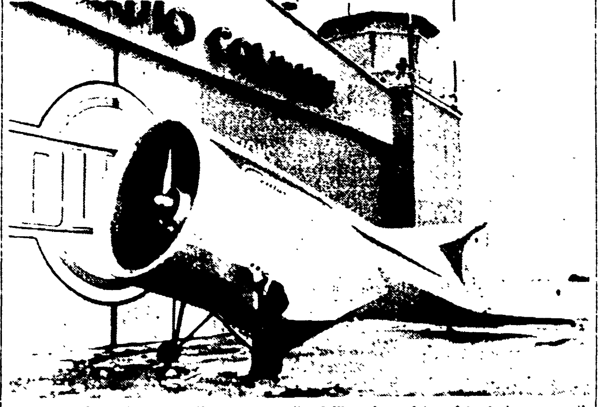
CEDAR RAPIDS (Iowa) — Il primo modello dell'aerodine fotografato insieme con il suo progettista dottor Alexander Lippisch, fuori dei locali del laboratorio di ricerche aeronautiche Collins nell'Iowa; l'aereo costruito per l'esercizio e l'aerodinamica, può innalzarsi verticalmente; il controllo di direzione è ottenuto da un timone convenzionale e da un elevatore. La cabina di pilotaggio (non visibile) sarà collocata dopo, sotto un baldacchino, nello stabilizzatore verticale. (Telefoto)
