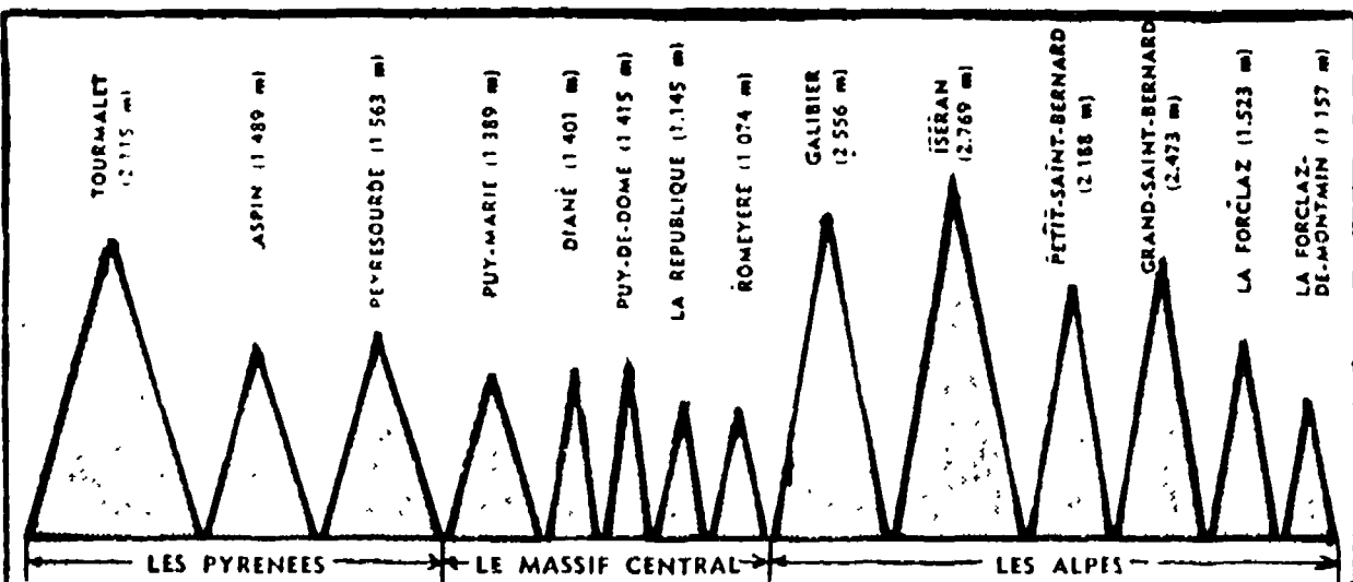
Il grafico altimetrico del tre gruppi di montagne: i Pirenei, il Massiccio Centrale e le Alpi
