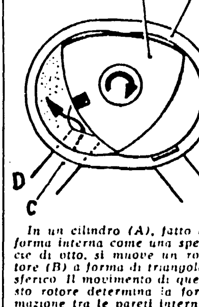
In un cilindro (A), fatto a forma interna come una specie di otto, si muove un rotore (B) a forma di triangolo sferico. Il movimento di questo rotore determina la formazione tra le pareti interne del cilindro A e il rotore B di camere a volume variabile nelle quali avvengono le normali quattro fasi di aspirazione, compressione, scoppio e scarico. La fase di aspirazione è rappresentata nel disegno sopra. L'aria entra attraverso il condotto (C) e la luce (D).
