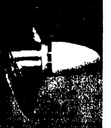
La particolarità di quest'elica, di origine americana, è quella di non avere le normali pale, ma, al loro posto, una sola superficie elicoidale che meglio delle pale, è adatta ad «avvitarsi» all'acqua...
