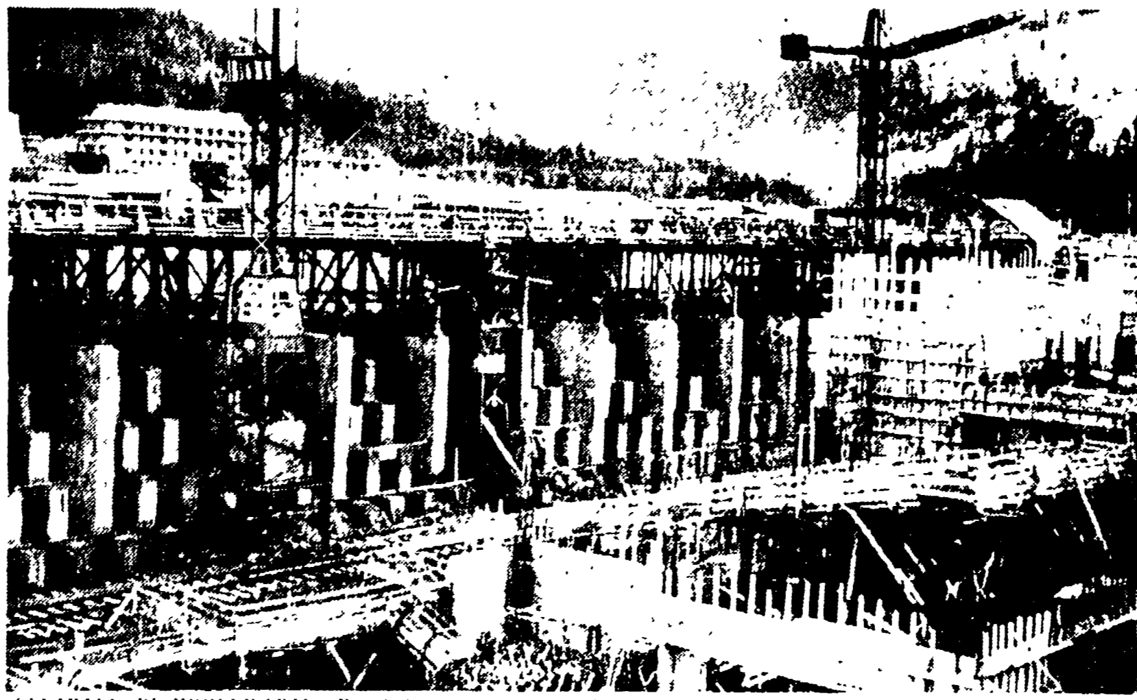
CENTRALE DI HOHNEWART (Repubblica democratica tedesca). La costruzione di questa grande centrale idroelettrica la più grande d'Europa procede rapidamente. I lavori sono in anticipo sul piano previsto. La centrale comincerà a fornire energia tra due anni.
