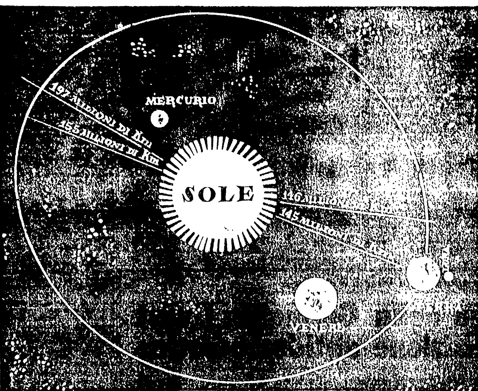
La posizione di alcuni pianeti (Terra, Venere, Mercurio) rispetto al Sole
