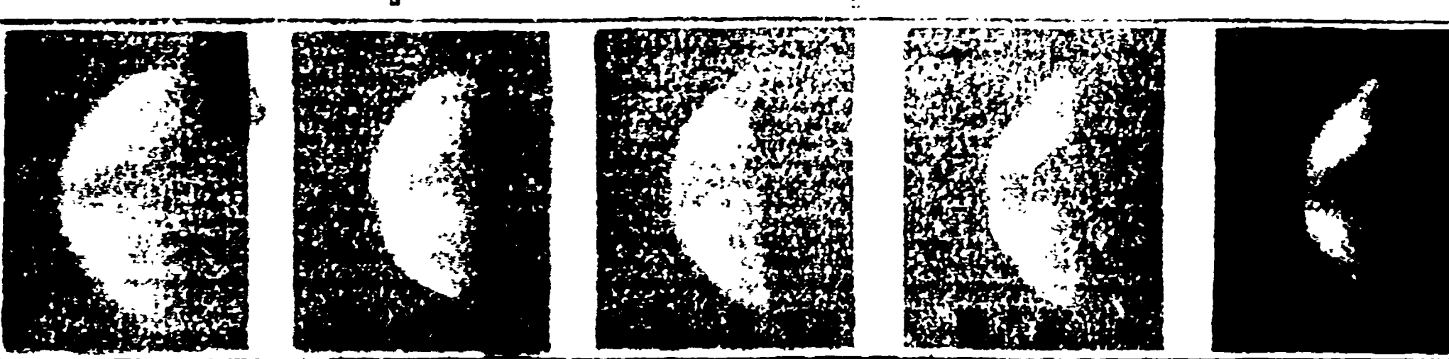
Alcune fasi del pianeta Venere fotografate da un grande telescopio americano nel 1937. Secondo i calcoli del sistema solare, Venere dista dal sole 108 milioni di Km, e compie la sua rivoluzione intorno ad esso in 224 giorni. Alla Terra non avviciniamo più di 40 milioni di Km, e la distanza minima è di 38 milioni di Km. Venere ha un diametro e un volume di pochissimo inferiori a quelli della
