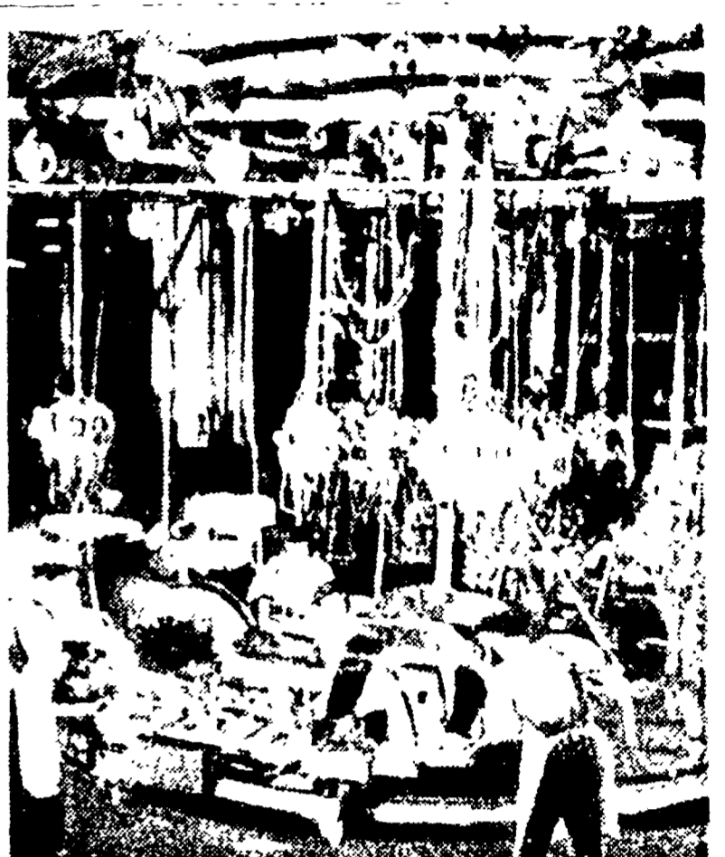
TORINO. MINATORI. Fabbrica volante con stazioni di saldatura per il fondo-scocca delle vetture scuo...
