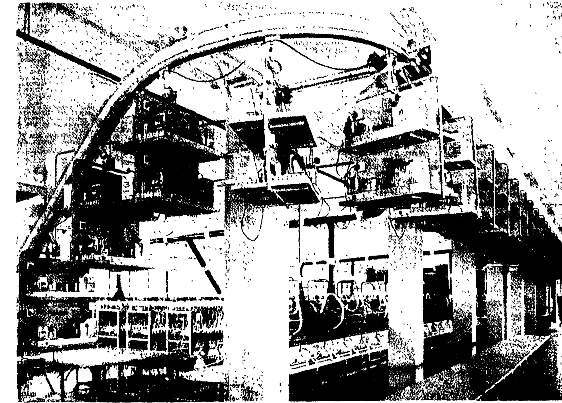
La modernissima catena di montaggio dei televisori «Majestic» un autentico gioiello della tecnica, perfetto come un orologio di gran marca.
