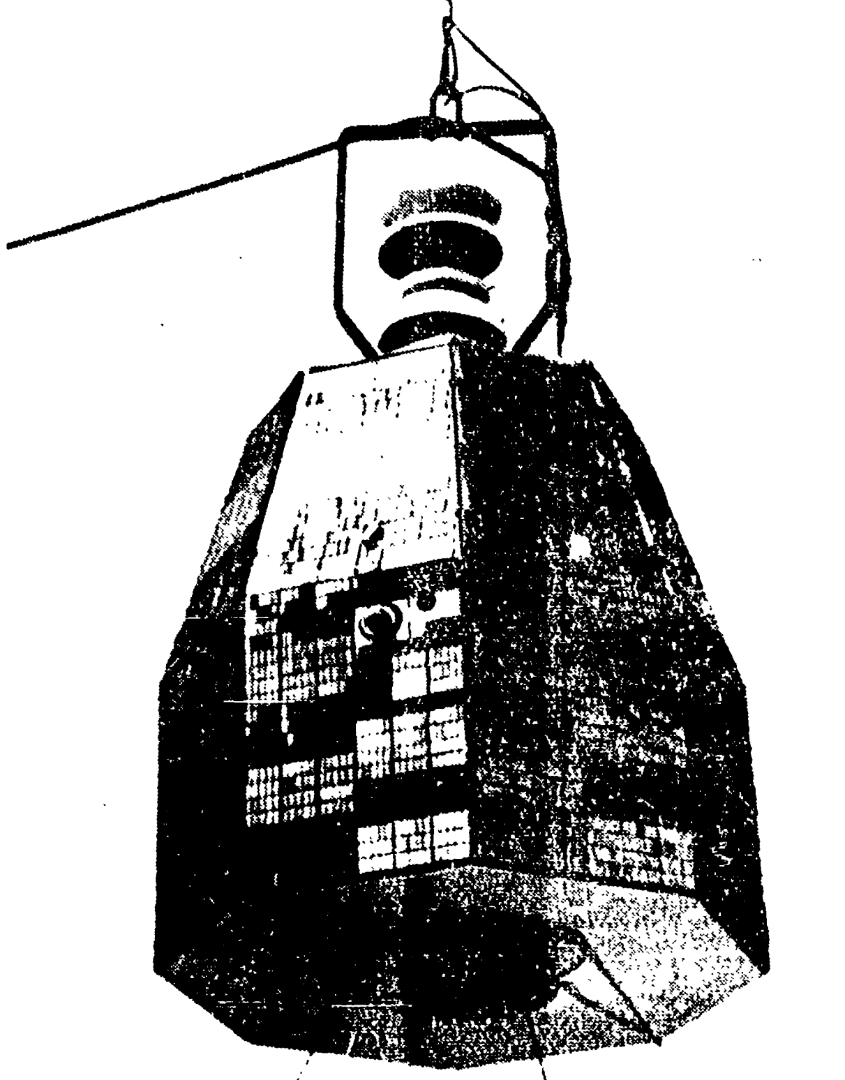
CAPE CANAVERAL — Il satellite Relay viene sollevato per essere sistemato in cima ad un razzo Thor-Delta
