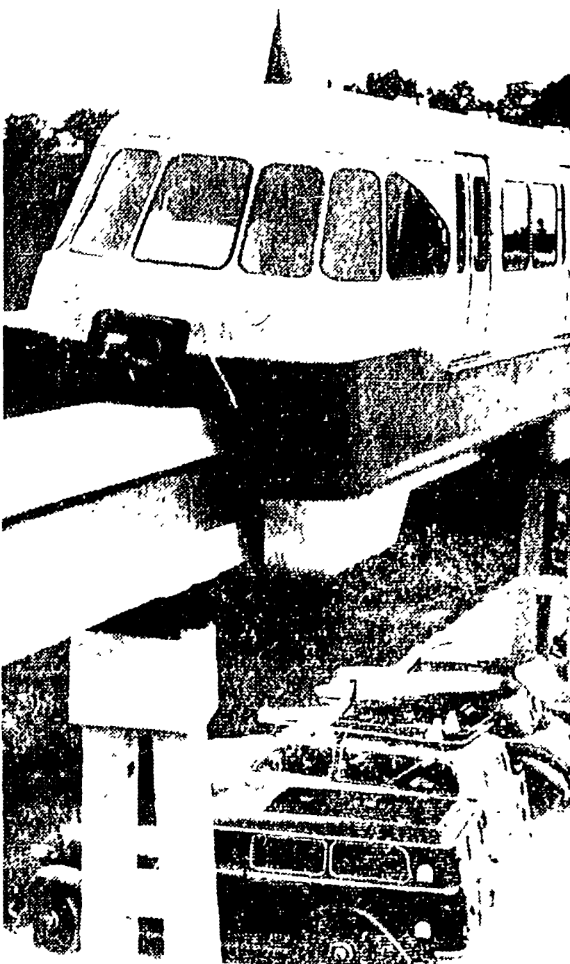
Un esempio di metrò aereo a Colonia, in Germania. Nel progetto allo studio in Campidoglio le vetture sono aggregate alla rotella del telaio invece che dal fondo come appare nella foto
