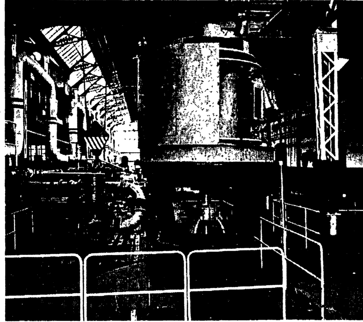
LA SPEZIA - Collaudo di una pompa di circolazione per centrale termoelettrica alla Termomeccanica Italiana.
