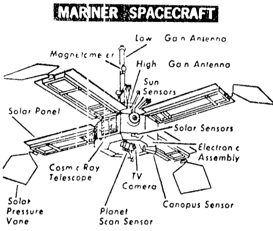
Il disegno schematico del Mariner IV
