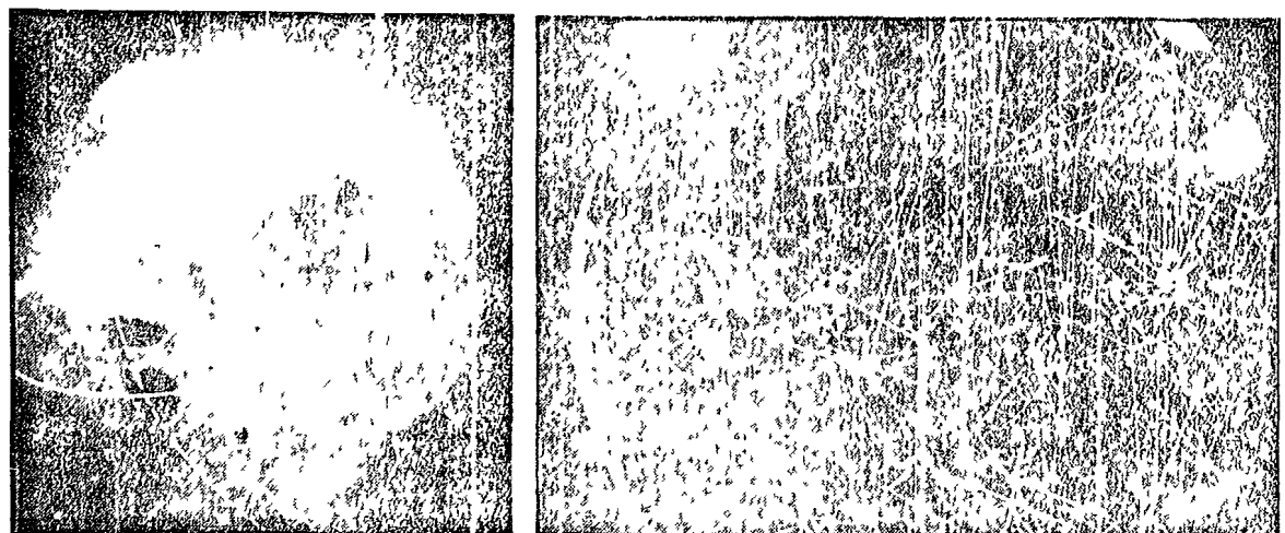
Una fotografia sovietica della «faccia nascosta» della Luna e (a destra) tracce di particelle nucleari generate dal bombardamento di atomi con protoni
