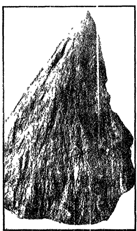
Cono di frammentazione trovato nel Sudafrica nell'astroblema di Vredford Ring. La sua lunghezza massima è di 10 centimetri
