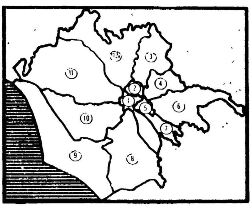
Le 12 circoscrizioni in cui dovrebbe essere suddiviso il territorio romano: 1) Centro Storico, Parco Appiense; 2) Parioli, Salaria, Nomentano; 3) Monte Mario; 4) Tiburtino; 5) Prenestino, Casilina; 6) Centocelle e le borgate all'Orto; 7) Tuscolano, Appio e Cinecittà; 8) Ostiense, Garbatella, EUR; 9) da Fregene a Castelgandolfo e nell'interzona sino a Casal Palocco; 10) Monteverde sino a Ponte Galeria; 11) Parioli, Aurelio, Trionfale, Primavalle; 12) dal Flaminio alla Cassia.
