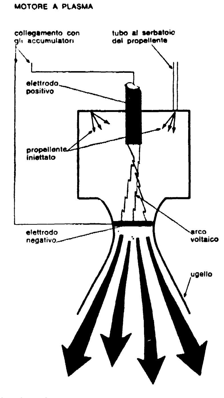
Lo schema di un motore a plasma
