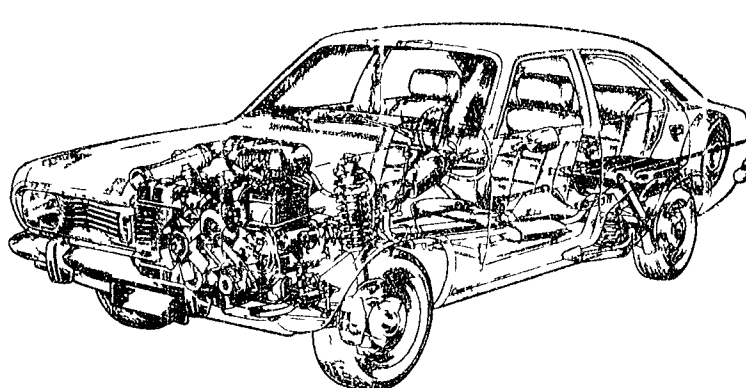
Vista in trasparenza delle nuove Chrysler. Gli organi meccanici sono disposti secondo lo schema classico.
