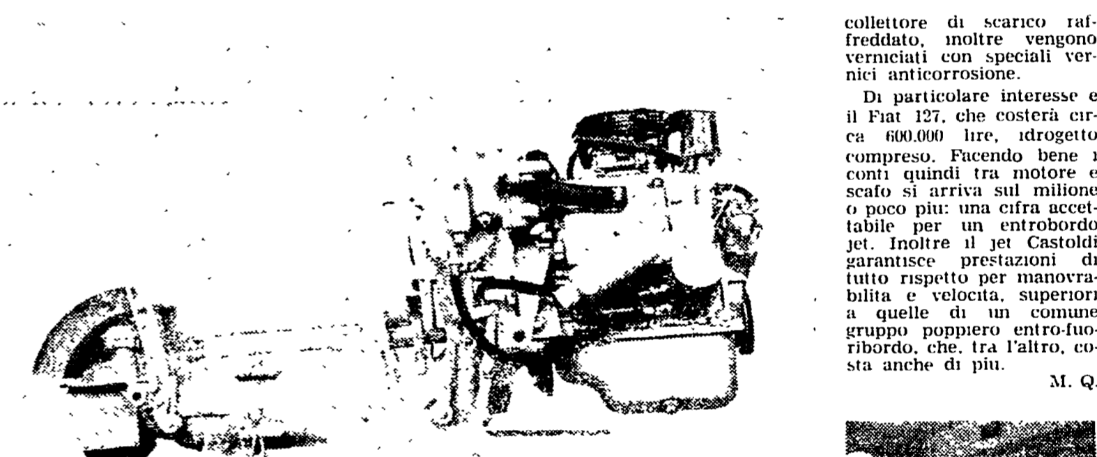
Il gruppo FIAT 127-Jet Castoldi Mod. 04, per complessivi 45 HP. La marinizzazione del motore viene eseguita dalla Castoldi con scambiatore di calore a circuito chiuso.
