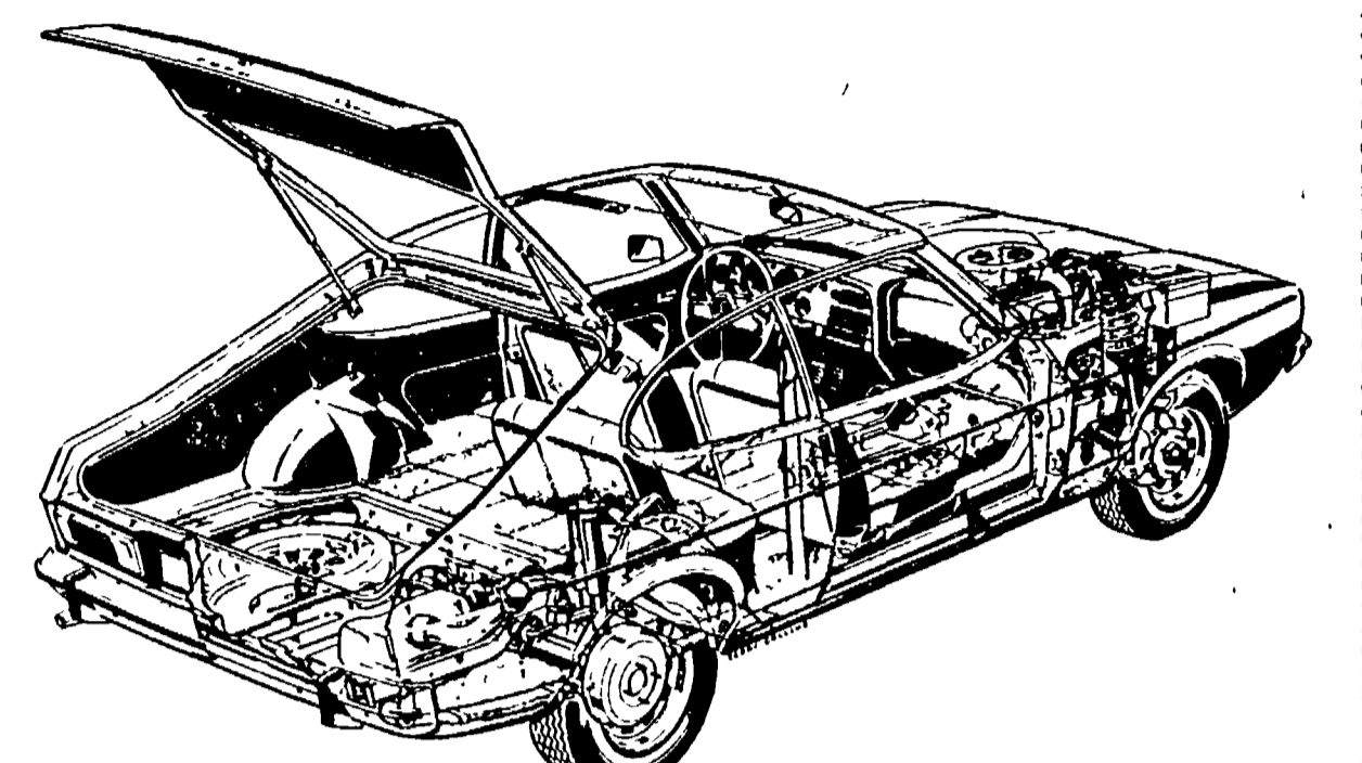
La Ford Capri II vista in trasparenza. Nel disegno si nota lo spazio a disposizione dei bagagli quando uno solo dei sedili posteriori è abbattuto.
