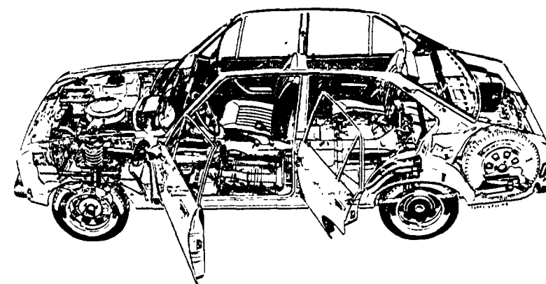
La nuova Ford «Escort» vista in trasparenza. Nel disegno in alto un particolare delle sospensioni posteriori modificate...
