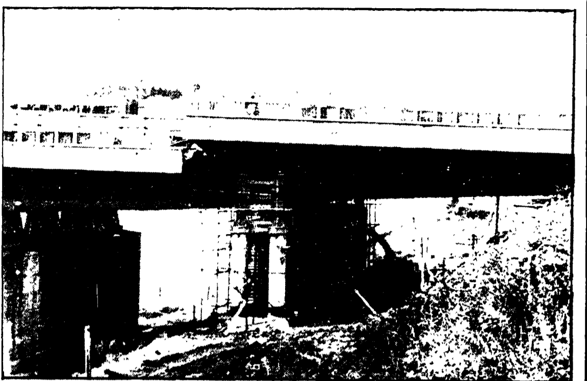
UN GIGANTESCO «CRICK» PER SALVARE IL PONTE. Con un gigantesco «crick», è stata sollevata una vata di oltre un metro una «fetta» di Ponte Marconi, a Roma, per rinforzare le strutture che hanno dato segni di cedimento. La stessa operazione si ripeterà nelle prossime settimane per altri due lastroni del ponte. Il traffico, comunque, scorre regolarmente: a essere tagliata e innalzata, infatti, è stata soltanto una corsia, mentre nell'altra le auto hanno via libera
