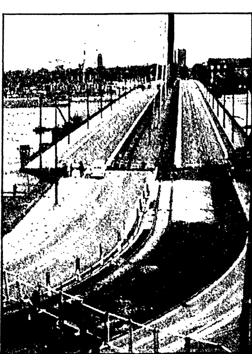
TRASLOCO DI UN PONTE. Il ponte sul Reno e Oberkassel è stato tagliato per essere trasferito a valle...
