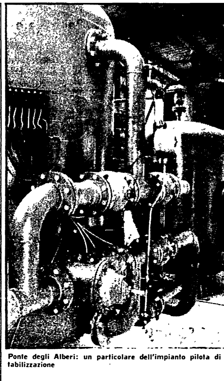
Ponte degli Alberi: un particolare dell'impianto pilota di potabilizzazione
