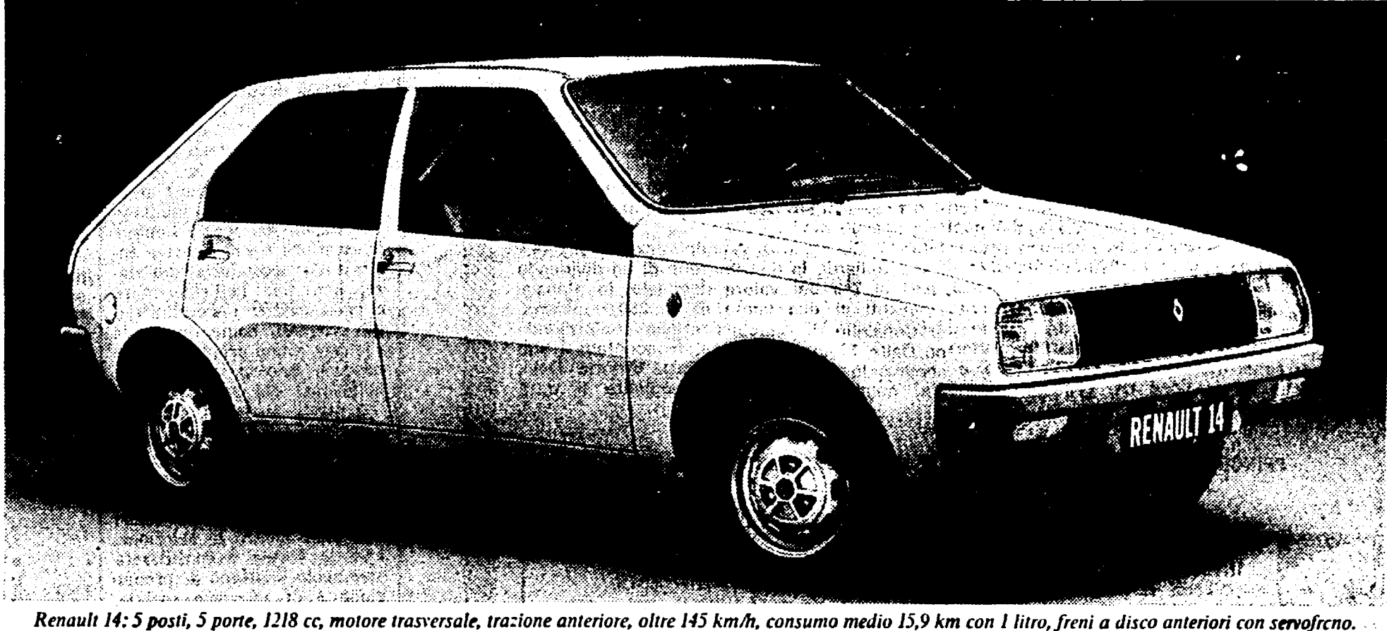
Renault 14: 5 posti, 4 porte, 1218 cc, motore trasversale, trazione anteriore, oltre 145 km/h, consumo medio 15,9 km con 1 litro, freni a disco anteriori con servofreno.
