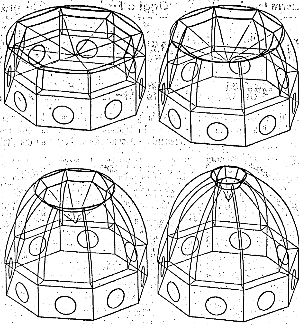
I vari stadi di costruzione di Santa Maria del Fiore secondo l'ipotesi avanzata da alcuni studiosi fiorentini. (Disegni dell'istituto di costruzioni della facoltà di Architettura, Firenze 1977).
